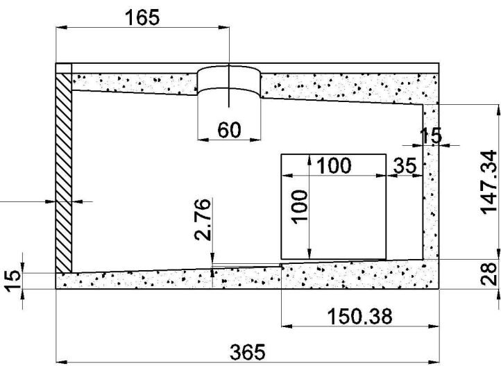
SECCIÓN A-A
