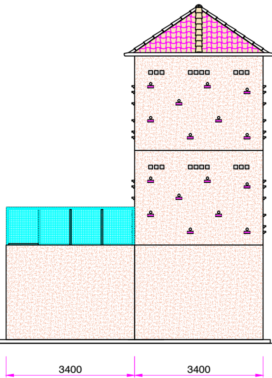
ALZADO 4
