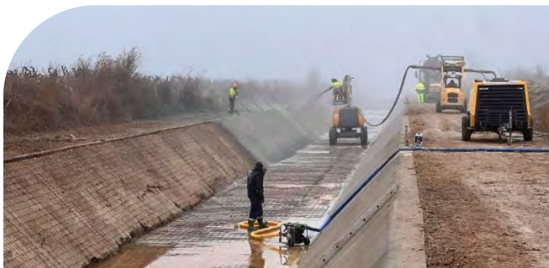
Gunitado del Canal de Aragón y Cataluña.
