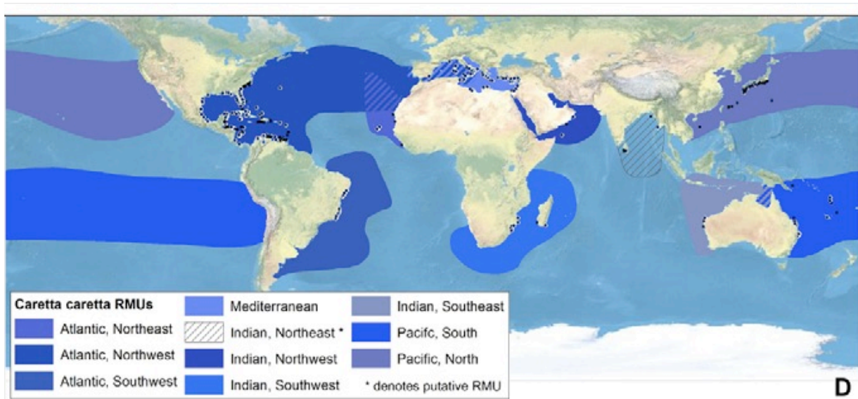
Figura 18. Unidades Regionales de Gestión para la tortuga boba. Tomado de Wallace et al., 2010. Se observan superposiciones de RMU en el Atlántico oriental y el Mediterráneo. Modificado de Wallace et al., 2010.
