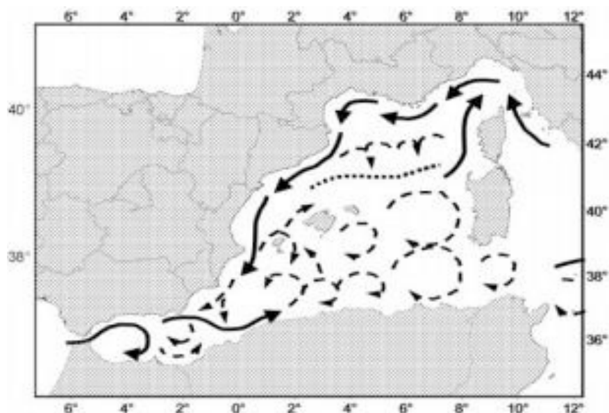
Figura 19. Patrón de corrientes superficiales para el Mediterráneo español. Se puede observar la corriente argelina (líneas discontinuas) y la corriente norte (líneas continuas), (Cardona et al., 2005).
