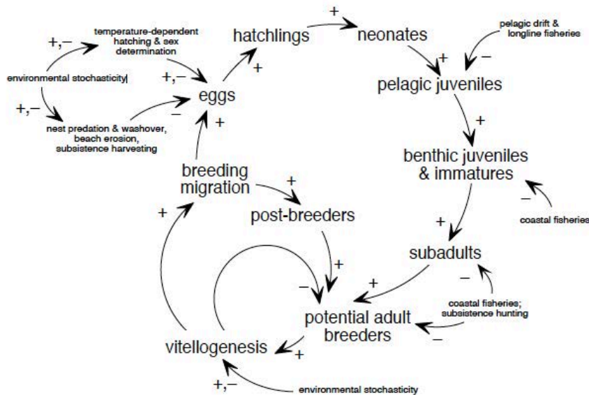
Figura 22 Ciclo de vida de la tortuga laúd
