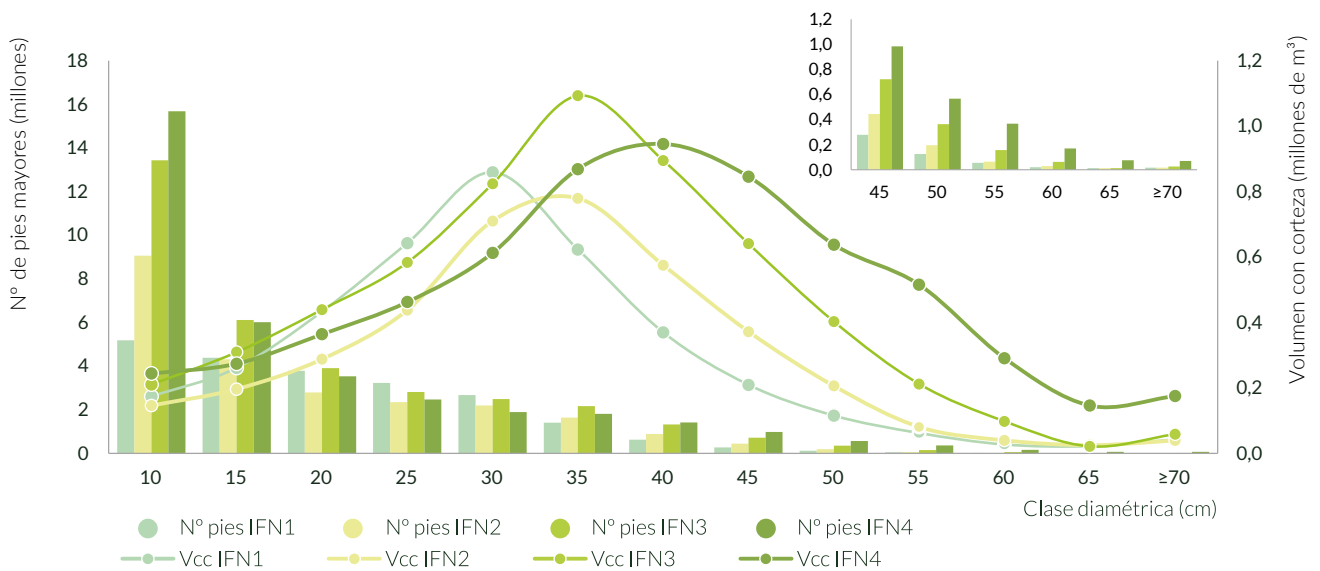
EVOLUCIÓN DE LAS EXISTENCIAS POR CLASE DIAMÉTRICA
