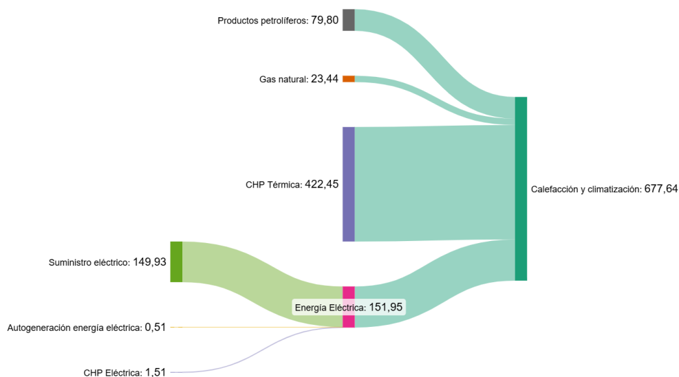
Figura 35. Distribución del consumo según fuentes de energía de la calefacción y climatización (GWh) en 2021.
