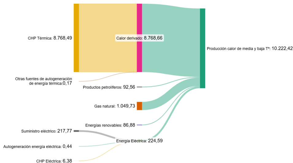
Figura 31. Distribución del consumo según fuentes de energía de la producción de calor de media y baja temperatura (GWh) en 2021.
