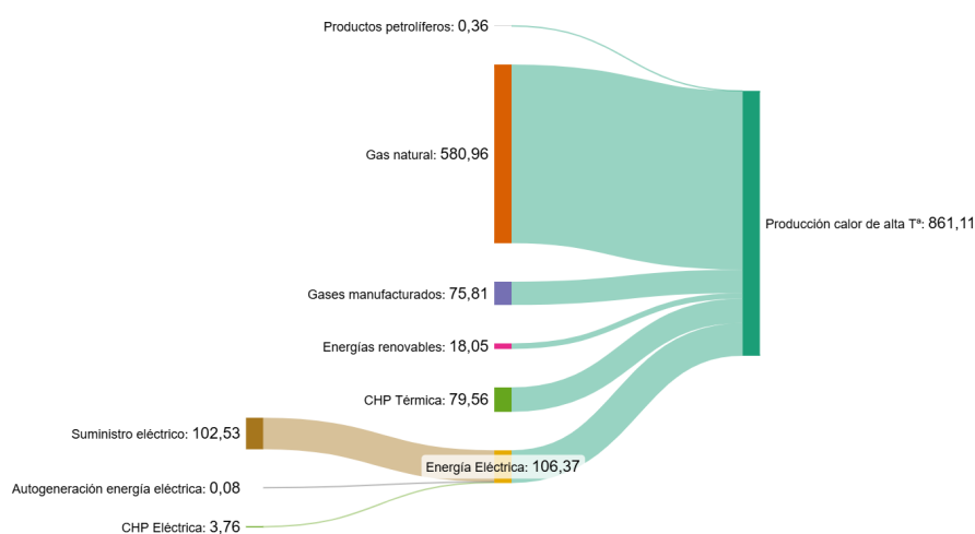
Figura 30. Distribución del consumo según fuentes de energía de la producción de calor de alta temperatura (GWh) en 2021.
