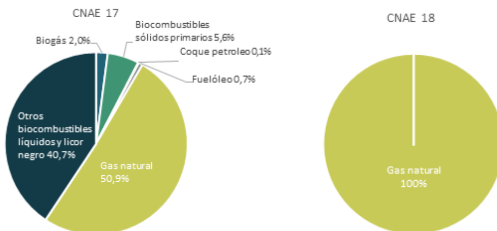
Figura 25. Distribución del consumo de combustibles en cogeneración para producción térmica por CNAE.
