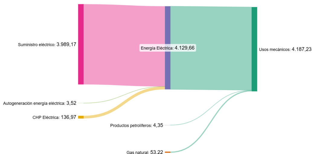
Figura 33. Distribución del consumo según fuentes de energía de los usos mecánicos (GWh) en 2021.
