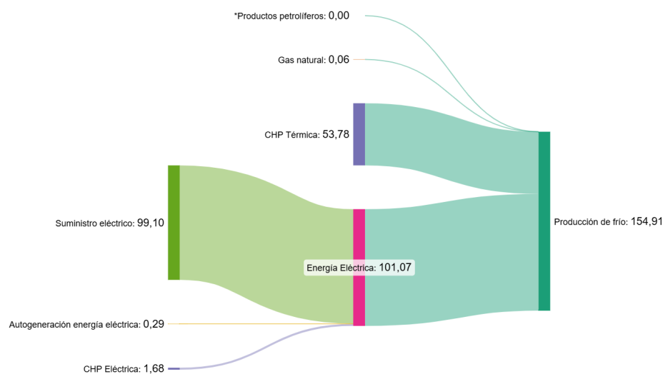
Figura 32. Distribución del consumo según fuentes de energía de la producción de frío (GWh) en 2021.
