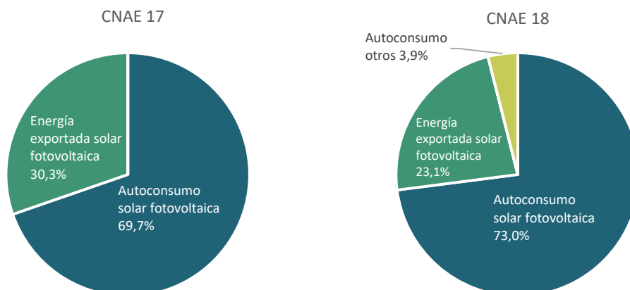
Figura 27. Distribución de energía eléctrica procedente de energías renovables y otros generadores por CNAE en 2021.
