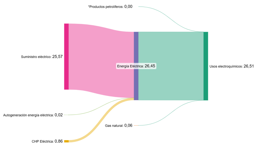
Figura 34. Distribución del consumo según fuentes de energía de los usos electroquímicos (GWh) en 2021.
