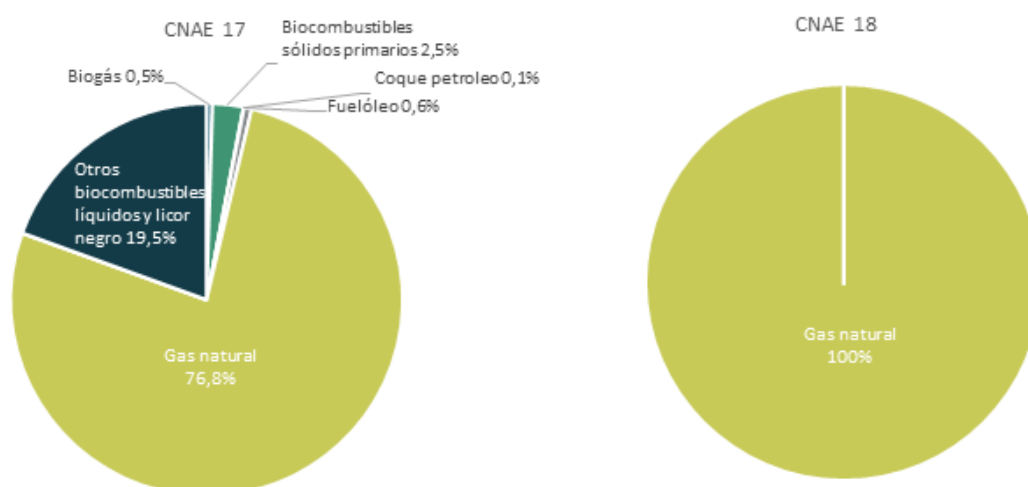
Figura 26. Distribución del consumo de combustibles en cogeneración para producción eléctrica por CNAE.
