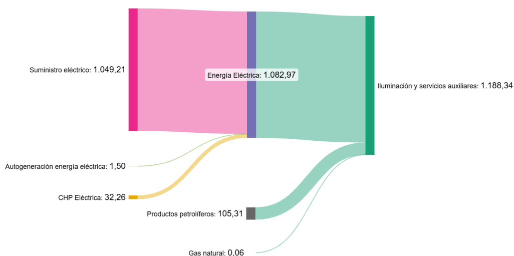
Figura 36. Distribución del consumo según fuentes de energía de la iluminación y sistemas auxiliares (GWh) en 2021.
