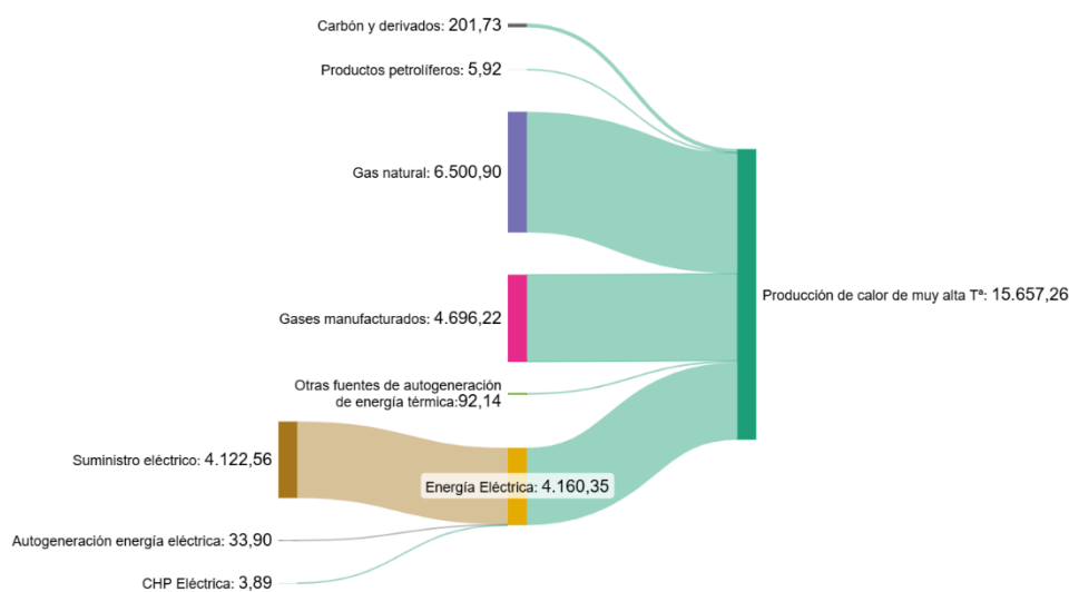
Figura 19. Distribución del consumo según fuentes de energía de la producción de calor de muy alta temperatura (GWh) en 2021.
