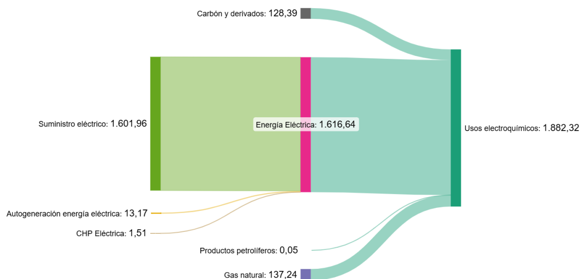
Figura 24. Distribución del consumo según fuentes de energía de los usos electroquímicos (GWh) en 2021.
