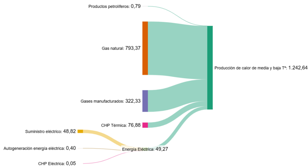
Figura 21. Distribución del consumo según fuentes de energía de la producción de calor de media y baja temperatura (GWh) en 2021.
