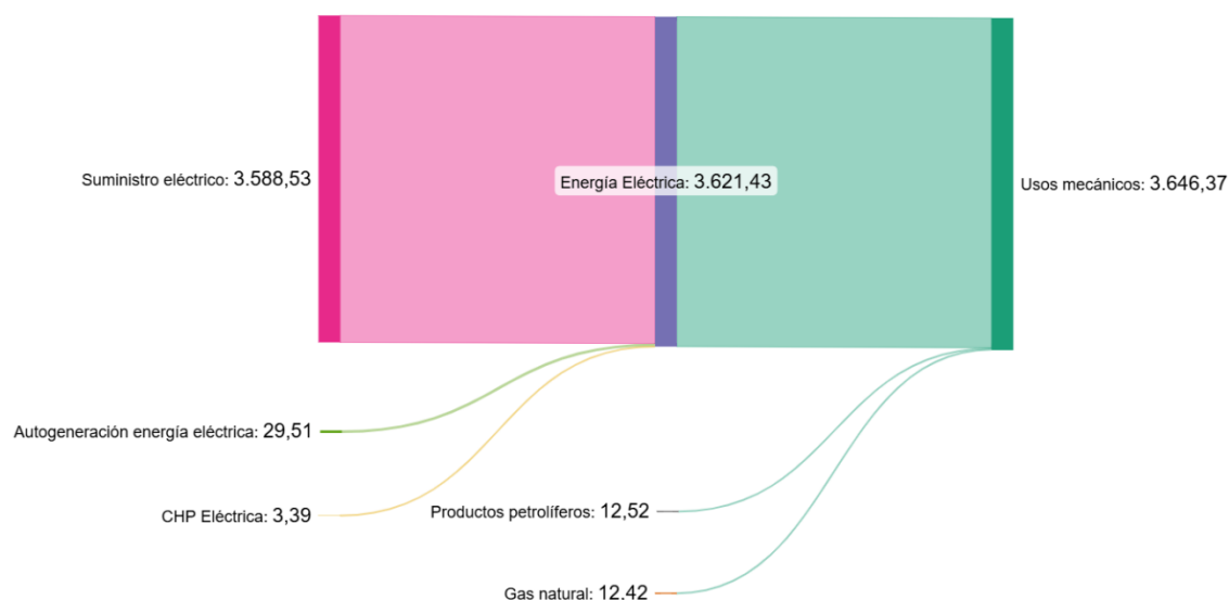
Figura 23. Distribución del consumo según fuentes de energía de los usos mecánicos (GWh) en 2021.
