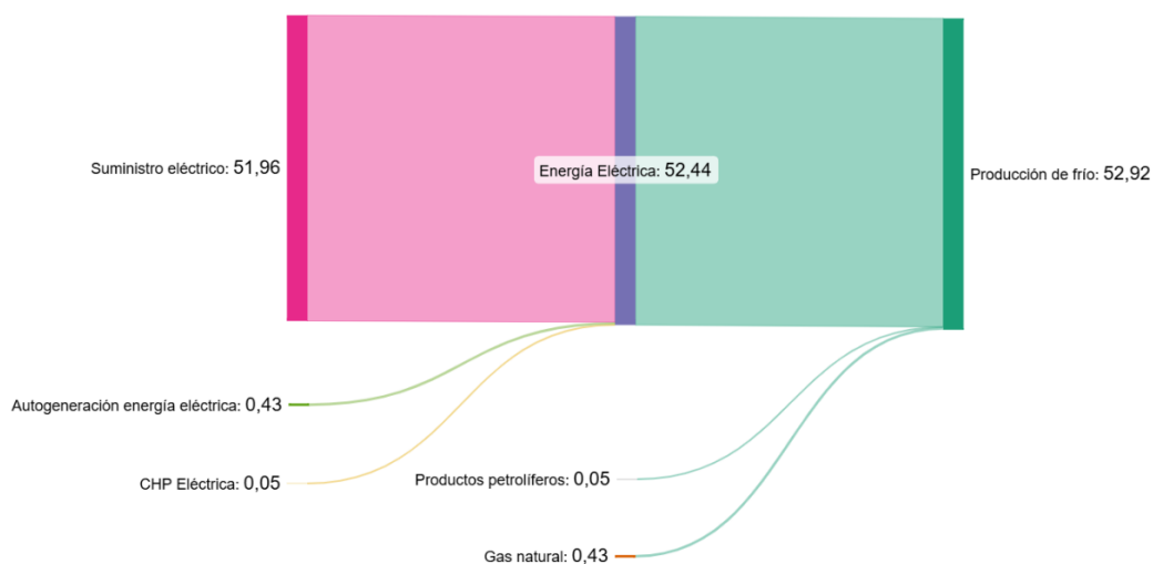
Figura 22. Distribución del consumo según fuentes de energía de la producción de frío (GWh) en 2021.
