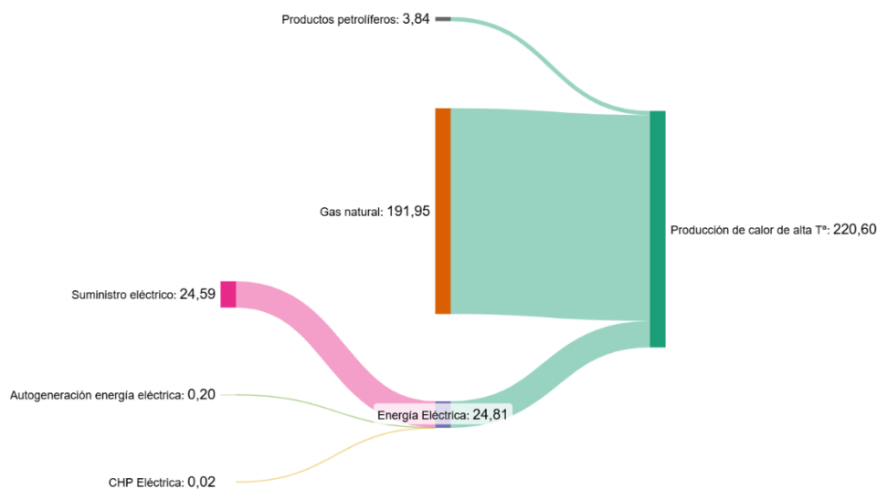
Figura 20. Distribución del consumo según fuentes de energía de la producción de calor de alta temperatura (GWh) en 2021.
