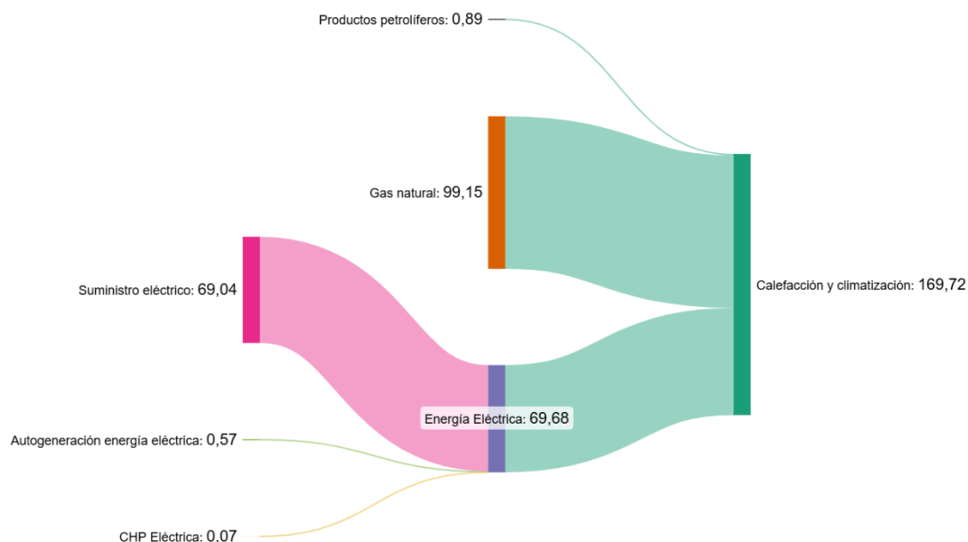
Figura 25. Distribución del consumo según fuentes de energía de la calefacción y climatización (GWh) en 2021.
