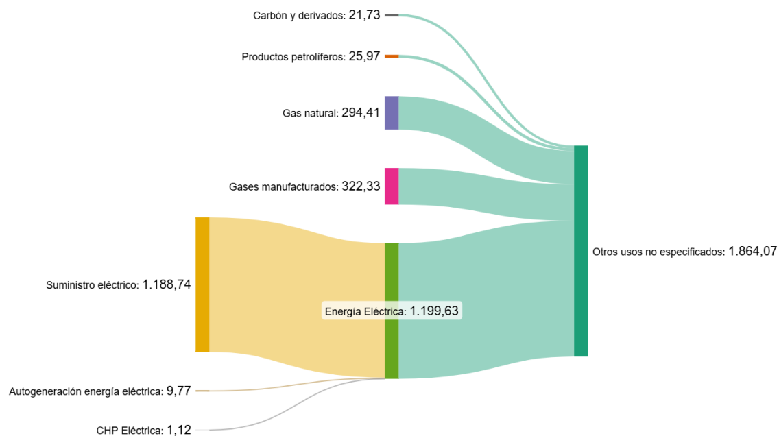
Figura 27. Distribución del consumo según fuentes de energía de otros usos no especificados (GWh) en 2021.
