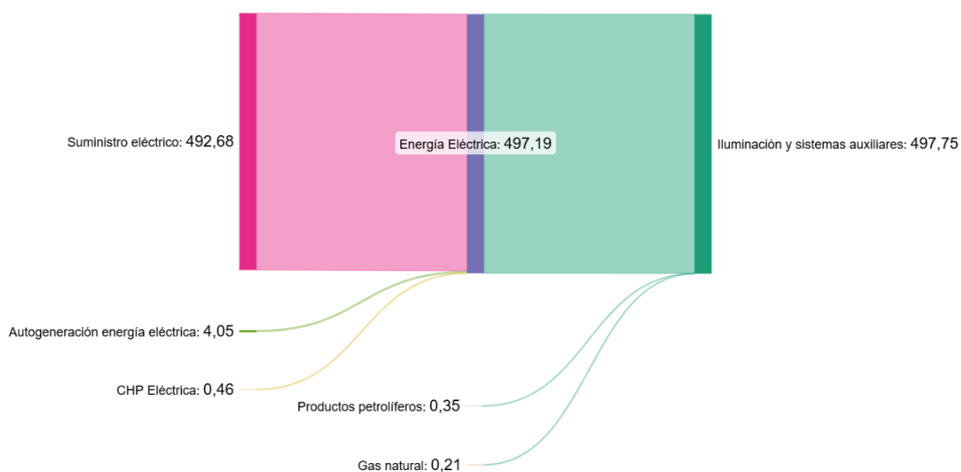
Figura 26. Distribución del consumo según fuentes de energía de la iluminación y sistemas auxiliares (GWh) en 2021.
