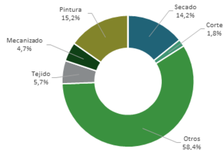
Procesos alimentados por combustibles y otras fuentes distintas de la electricidad
