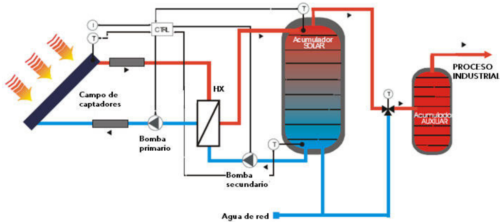
Figura 29: Esquema de principio tipo para calor de procesos con solar. Conexión en serie
