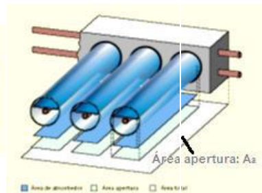
Figura 15: Área apertura tubos de vacío
