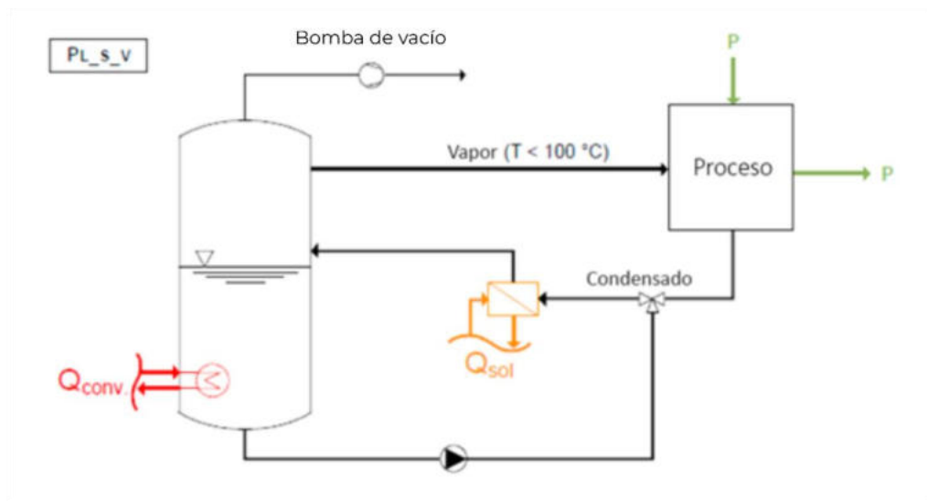
Figura 37: Acoplamiento en paralelo: Solar para la producción directa de vapor ( T < 100\text{ °C} ) para el proceso http://www.zero-emissions.at/index.php?title=EFFICIENCY_FINDER
