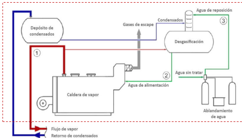
Figura 33: Ejemplo de proceso industrial de producción de vapor
