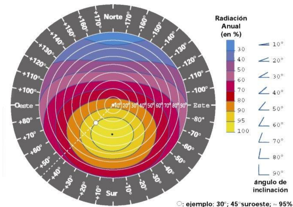
Figura 4: Relación entre la radiación global disponible sobre la apertura de un captador estacionario con una determinada inclinación sobre la horizontal y una determinada orientación y la radiación máxima posible.
