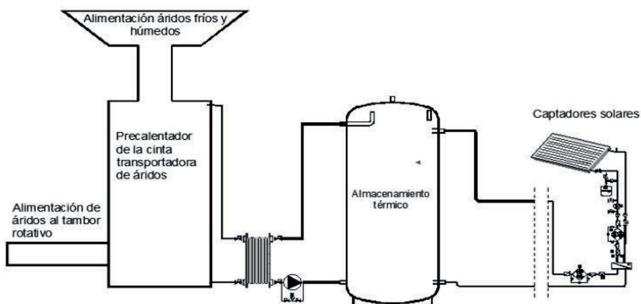
Esquema simplificado de la integración de la instalación solar
