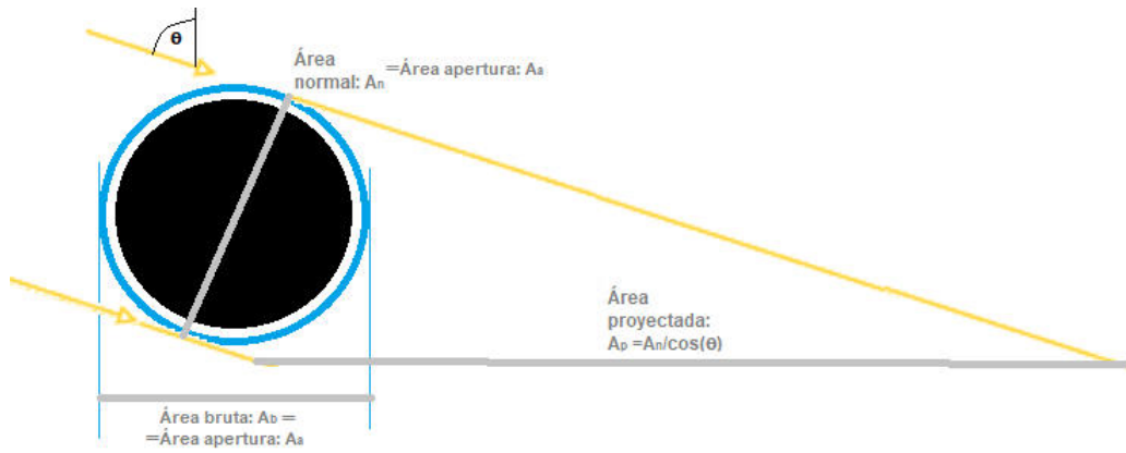
Figura 21: Área que ilumina el absorbente para un ángulo de incidencia \theta , proyectada sobre el plano que define el área de apertura
