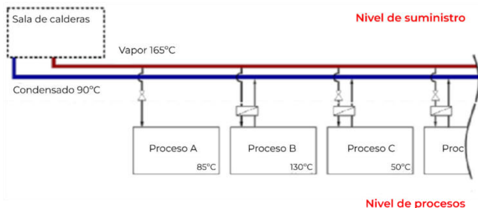
Figura 26: Distribución del calor a los diversos procesos
