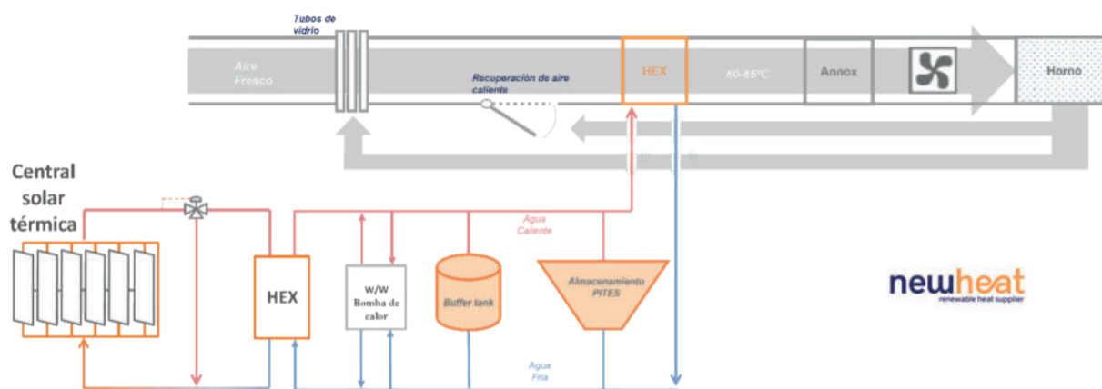
Esquema simplificado de integración del calor renovable en el proceso industrial (© Newheat)
