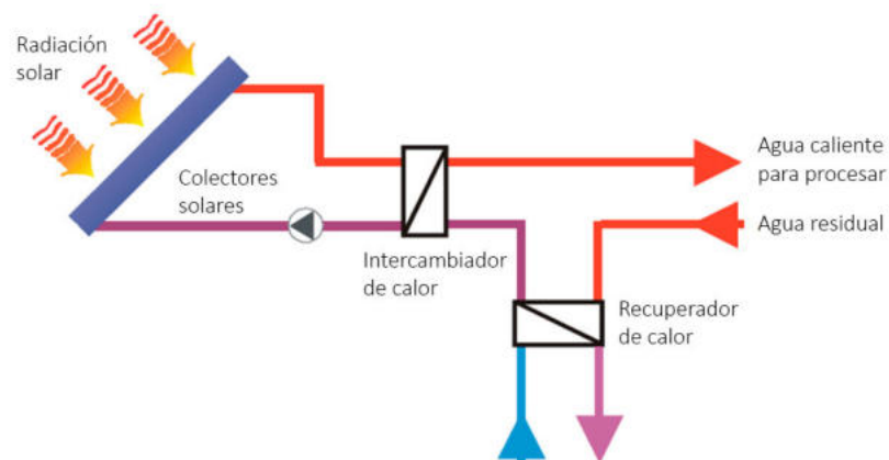
Figura 31 Hibridación con sistemas de recuperación de calor
