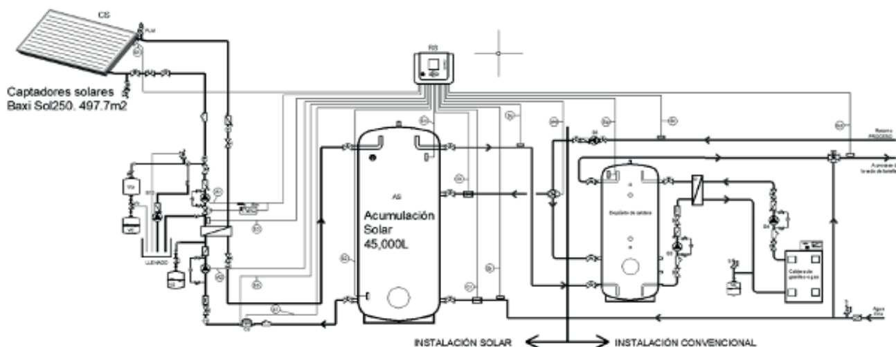
Esquema simplificado de la integración de la instalación solar
