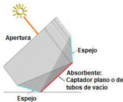
Figura 19: Área de apertura de un TC-FTC con 2 espejos
