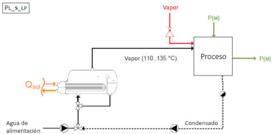
Figura 38: Acoplamiento en paralelo: Solar para la producción indirecta de vapor ( T > 100\text{ °C} ) para el proceso http://www.zero-emissions.at/index.php?title=EFFICIENCY_FINDER
