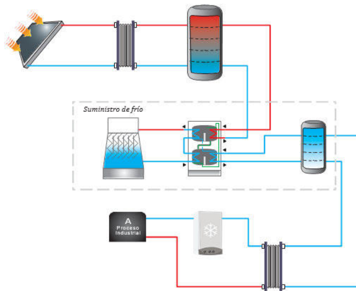
Figura 32: Esquema para la producción de frío para un proceso industrial
