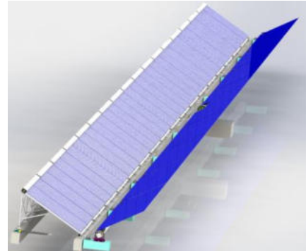
Figura 10: Captador solar fijo con concentrador externo acoplado: 1 espejo plano con seguimiento
