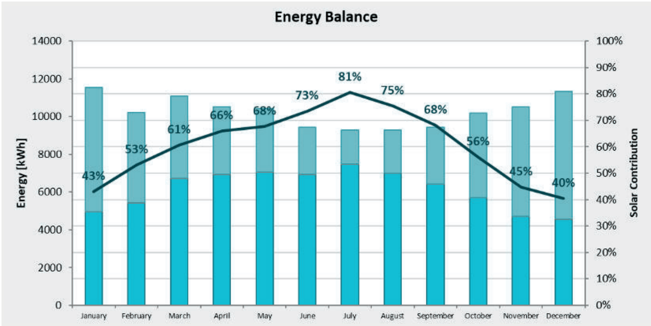
Perfiles mensuales de demanda y aporte solar
