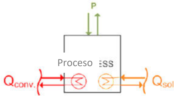
Figura 36: Acoplamiento en serie: Solar para el precalentamiento del retorno del proceso (Calentamiento indirecto con intercambiador interno) http://www.zero-emissions.at/index.php?title=EFFICIENCY_FINDER
