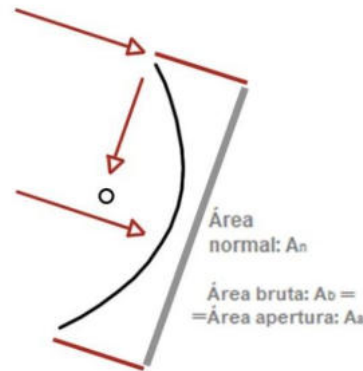
Figura 17: Área de apertura de un cilindro parabólico
