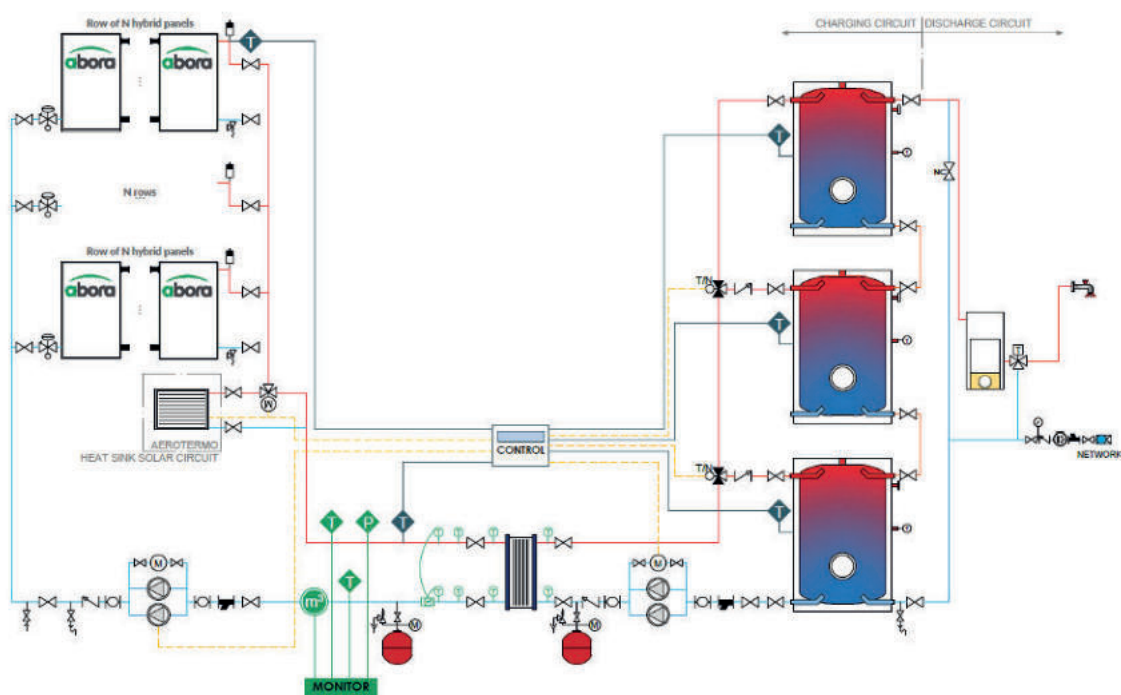
Esquema simplificado de la integración de la instalación solar
