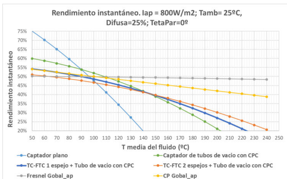
Figura 22: Rendimiento instantáneo, referido a la radiación global, de las tecnologías consideradas para un ángulo de incidencia nulo
