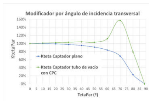
Figura 23: KtetaPar para captadores estacionarios
