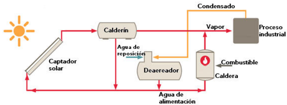
Figura 30 Esquema de principio tipo para calor de procesos con solar: Conexión en paralelo
