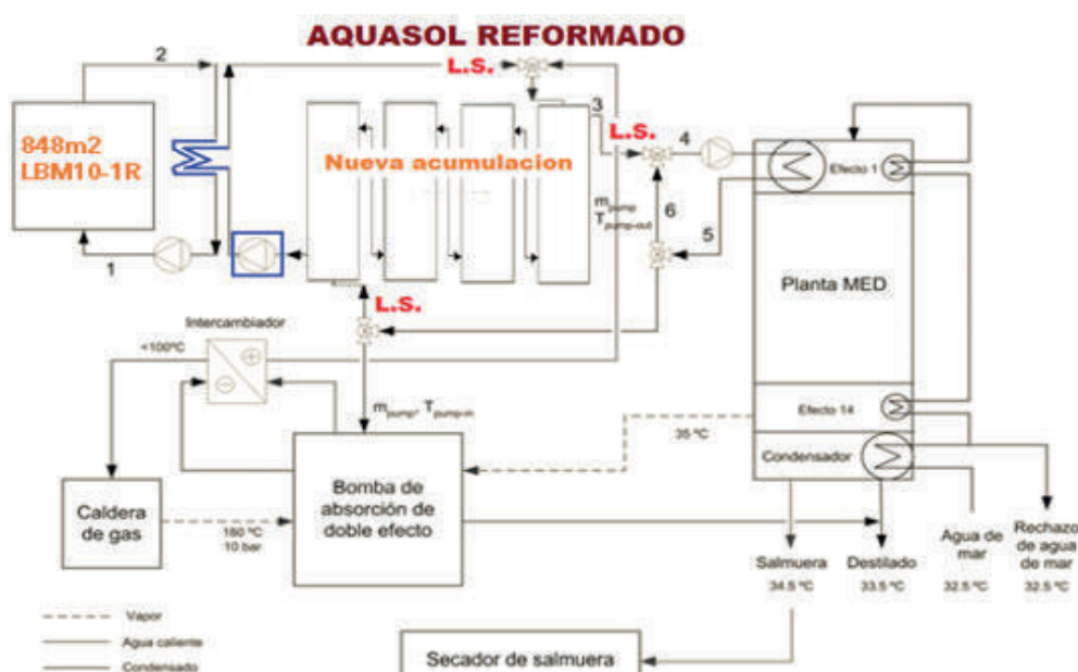
Esquema simplificado de la integración de la instalación solar
