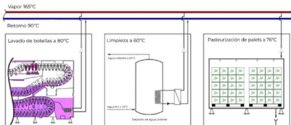
Figura 27: Ejemplo de reparto de calor a diversos procesos
