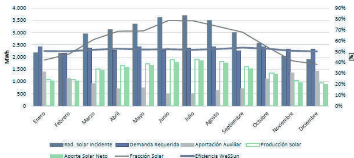
Perfiles mensuales de radiación solar disponible, demanda del secado de lodos, aporte solar neto, fracción solar y eficiencia solar
