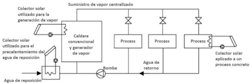
Figura 34: Opciones de acoplamiento solar en los procesos industriales
