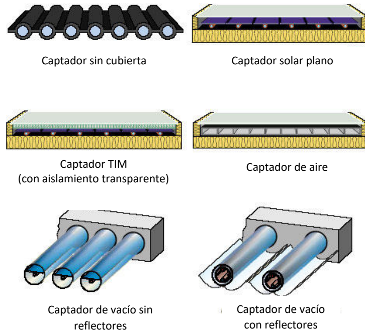
Figura 6: Captadores solares estacionarios
