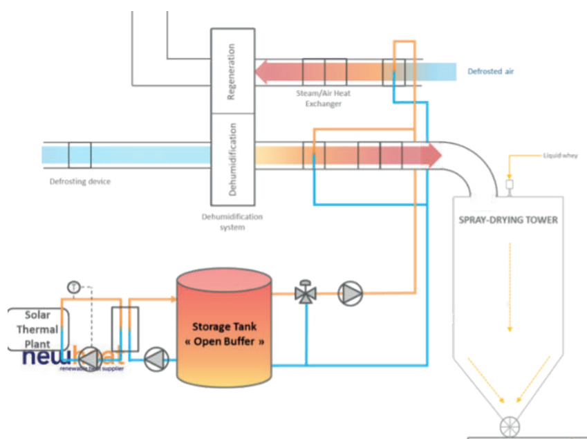
Esquema simplificado de integración del calor renovable en el proceso industrial (© Newheat)
