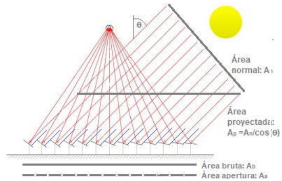
Figura 18: Área de apertura de un concentrador lineal Fresnel
