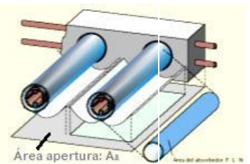
Figura 16: Área apertura tubos de vacío con reflector trasero
