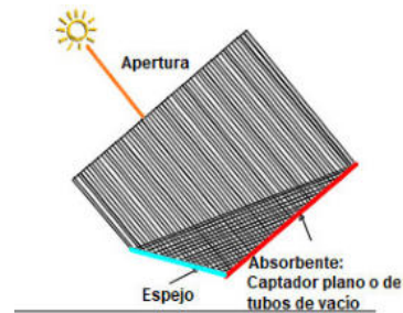
Figura 20: Área de apertura de un TC-FTC con 2 espejos
