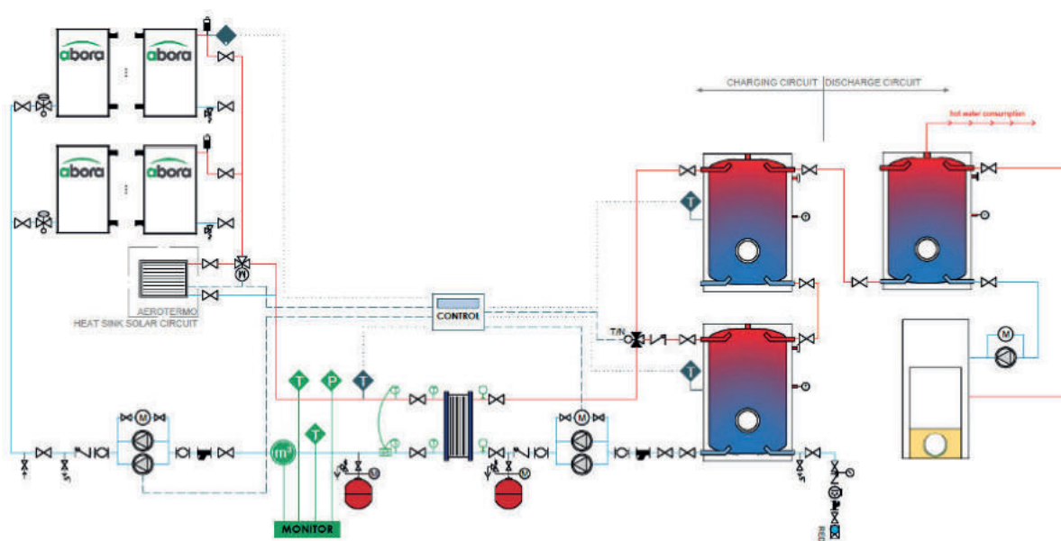
Esquema simplificado de la integración de la instalación solar
