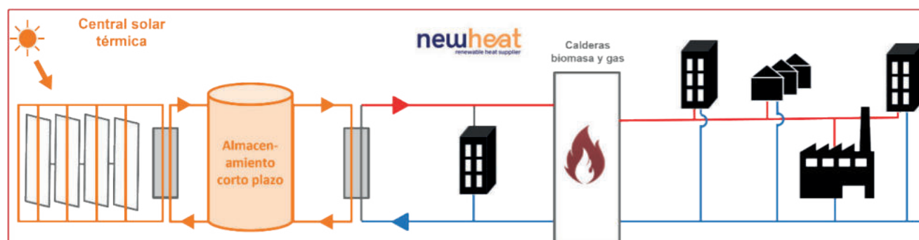
Esquema simplificado de integración del calor renovable en la red de calor urbana (© Newheat)
