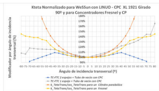
Figura 24: KtetaPar normalizado para captadores con seguimiento
