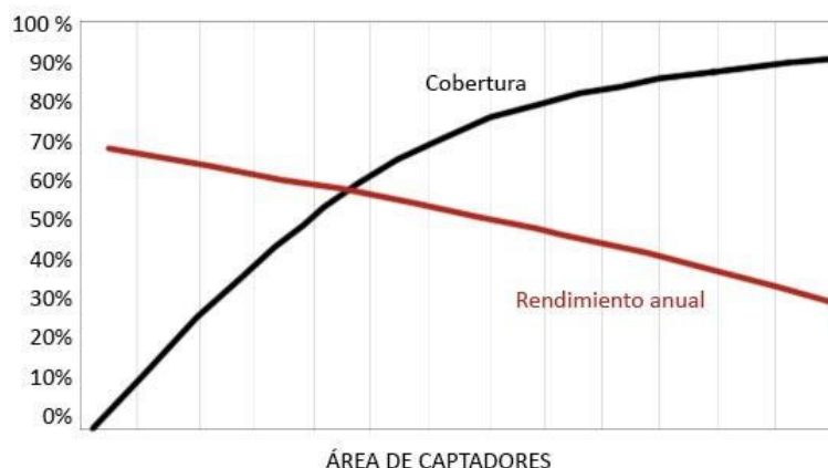
Figura 25: Rendimiento y cobertura solar anual
