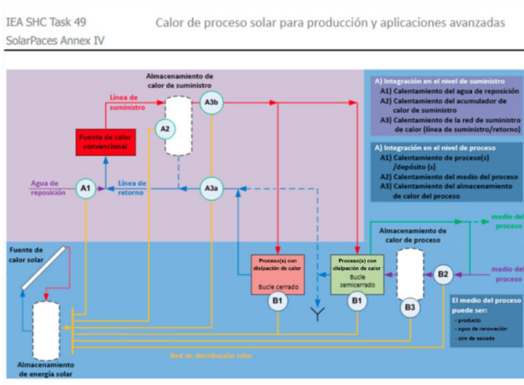
Figura 28 Posibilidades para la integración solar en el proceso (AEE INTEC, 2012)
