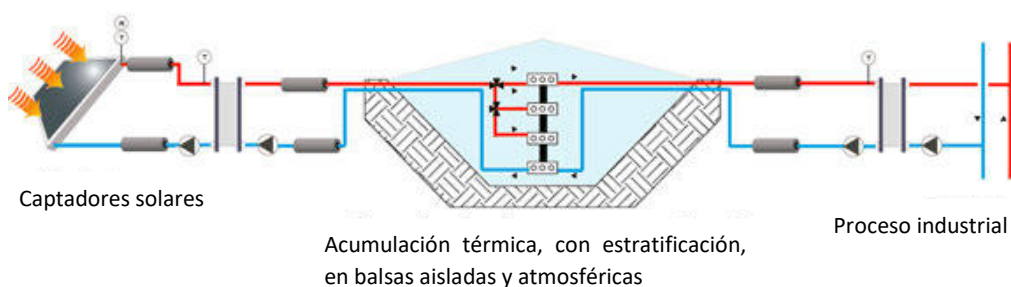
Figura 12: Acumulación solar para grandes volúmenes de acumulación a presión atmosférica
