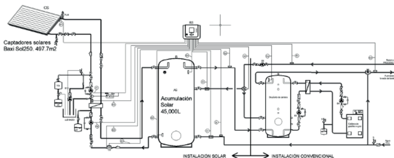
Esquema simplificado de la integración de la instalación solar
