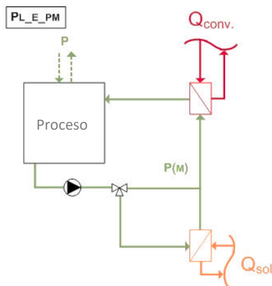
Figura 35; Acoplamiento en serie: Solar para el precalentamiento del retorno del proceso (Calentamiento indirecto con intercambiador externo) http://www.zero-emissions.at/index.php?title=EFFICIENCY_FINDER
