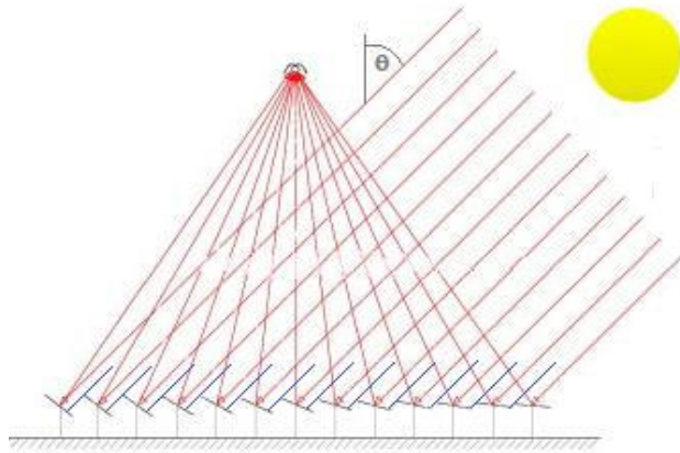
Figura 8: Concentrador Fresnel
