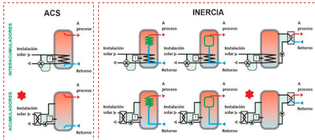
Figura 11: Tipologías de acumuladores solares presurizados
