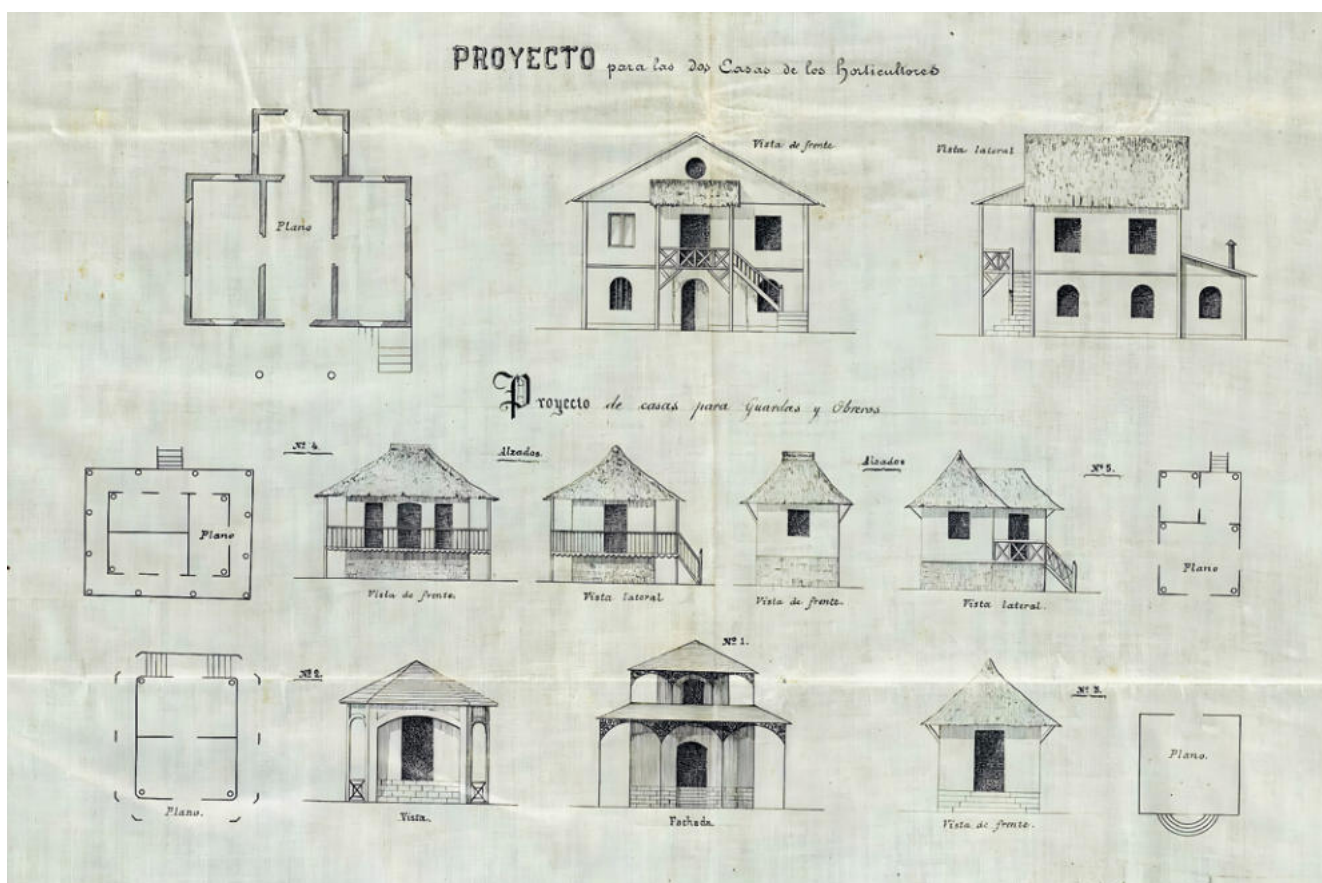
Fig. 19. Proyecto de casas para horticultores, guardas y alumnos obreros incluido en el proyecto de Jardín botánico firmado por Ramón Jordana el 27 de julio de 1877 (AHN. ULTRAMAR. MPD-5481).
