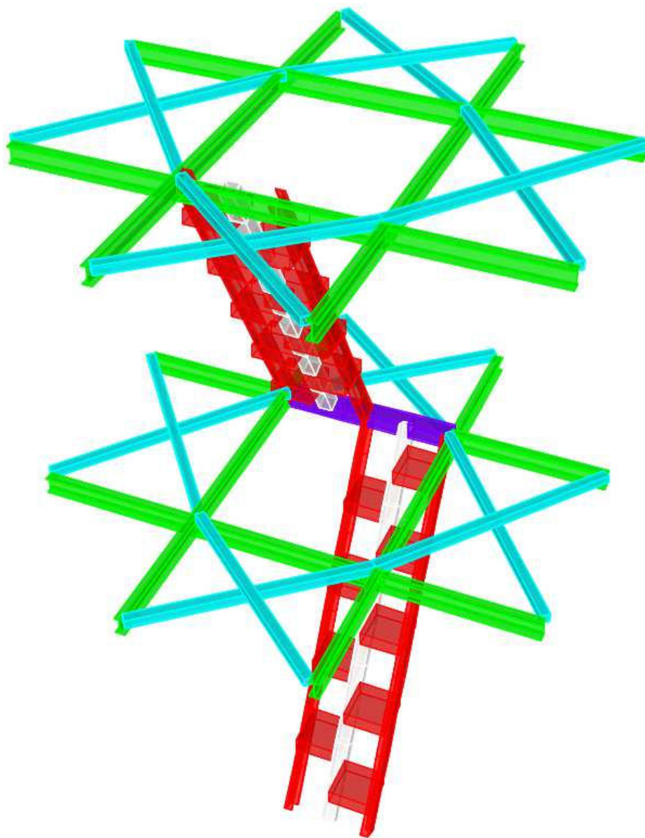
ESTRUCTURA INTERIOR NIVELES 1 y 2.
