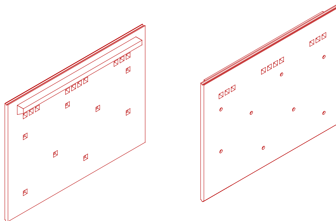
ALZADO DESDE INTERIOR
