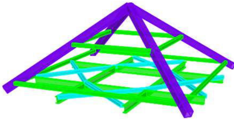
ESTRUCTURA INTERIOR CUBIERTA Y ARRIOSTRADO CABEZA SUPERIOR
