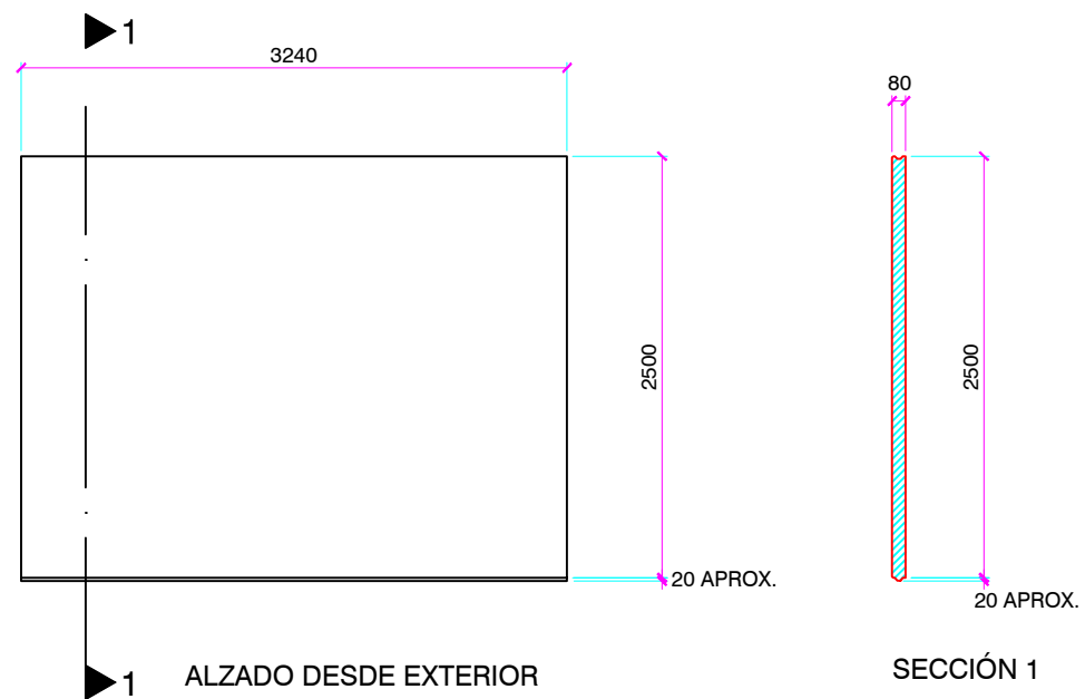
PANEL P3 PATIO (1 UNIDAD)
