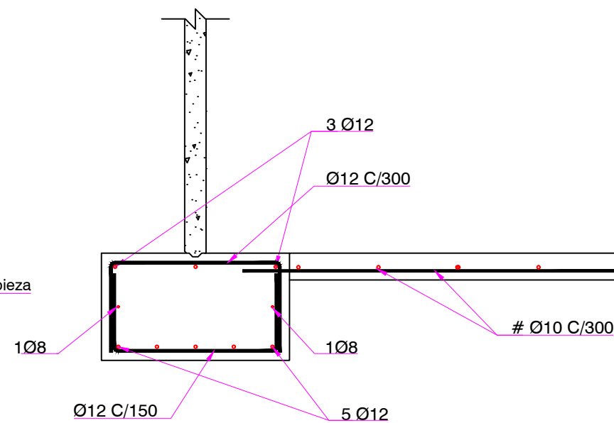
ZAPATA CORRIDA ESCALA 1:20 COTAS EN MILÍMETROS
