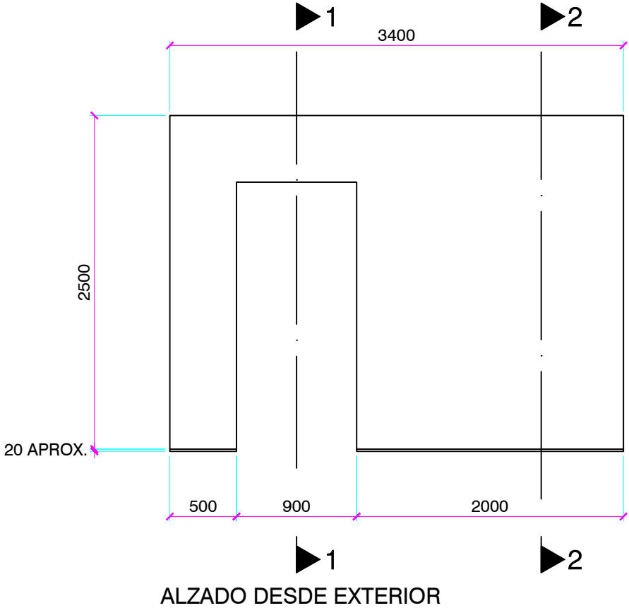
PANEL E.1 NIVEL 0. PATIO (1 UNIDAD)
