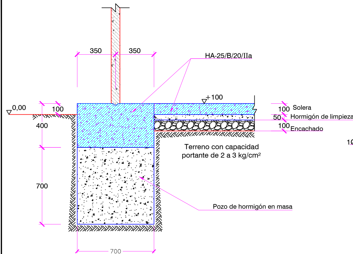
ZAPATA CORRIDA ESCALA 1:20 COTAS EN MILÍMETROS
