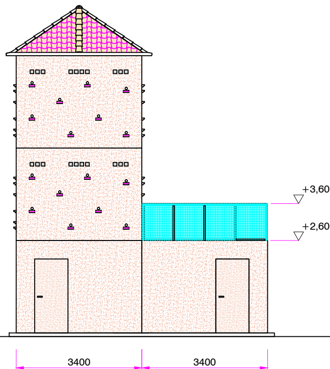
ALZADO 2
