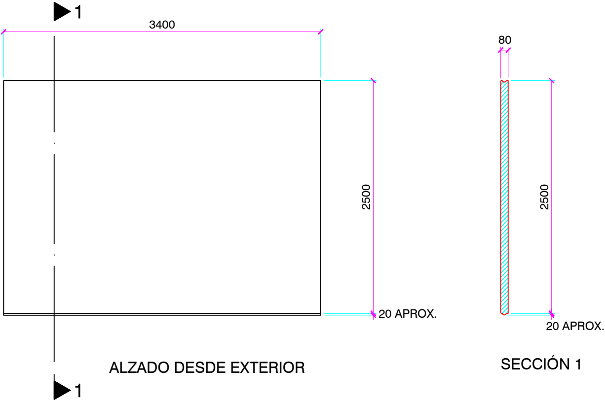
PANEL E.2 NIVEL 0 (1 UNIDAD)
