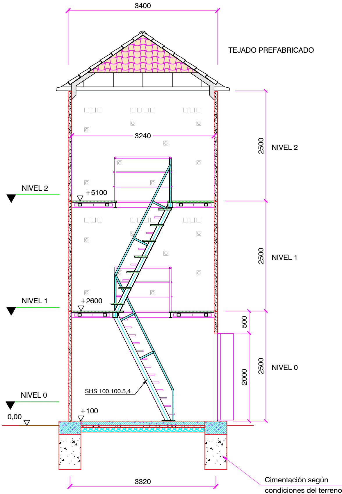
SECCIÓN-ALZADO B-B'
