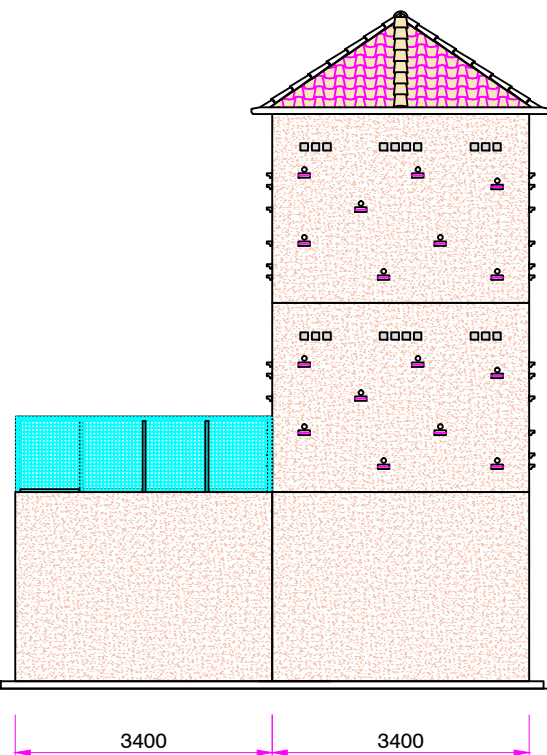
ALZADO 4
