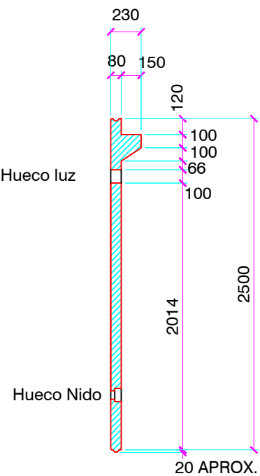
SECCIÓN 1
