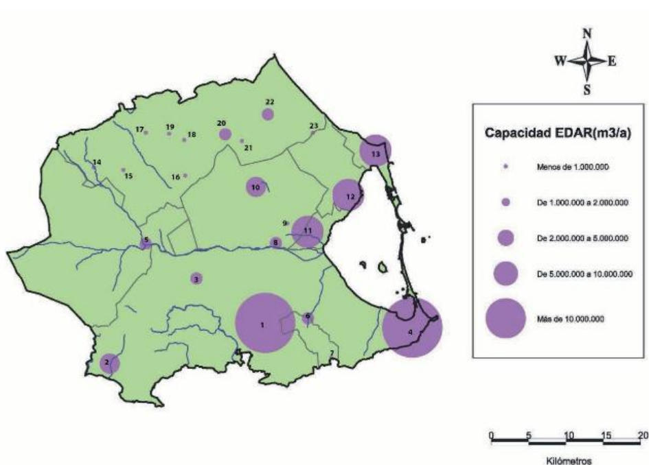
Figura 5.6. EDAR en la comarca Campo de Cartagena – Mar Menor. Fuente: elaboración propia con gvSIG a partir de datos de ESAMUR.
