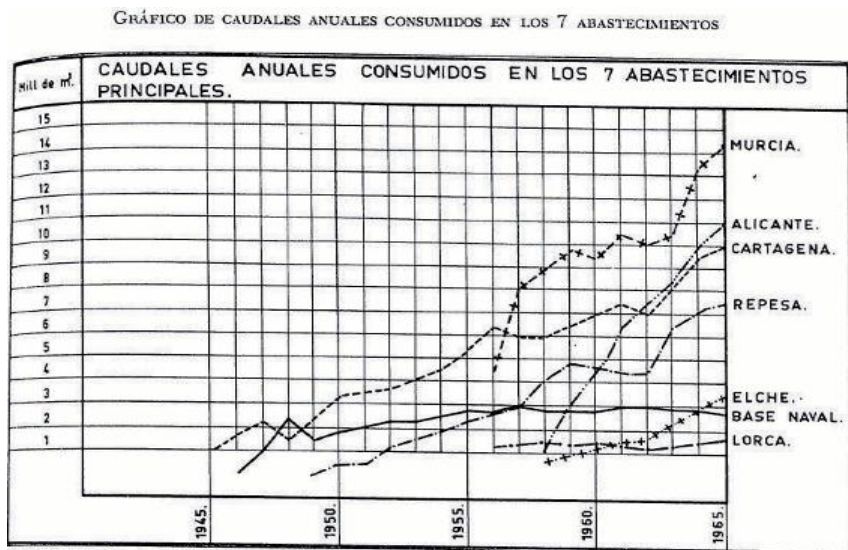
Figura 3.31. Gráfica de caudales anuales consumidos en los siete abastecimientos principales. Fuente: De la Cerda (1966).
