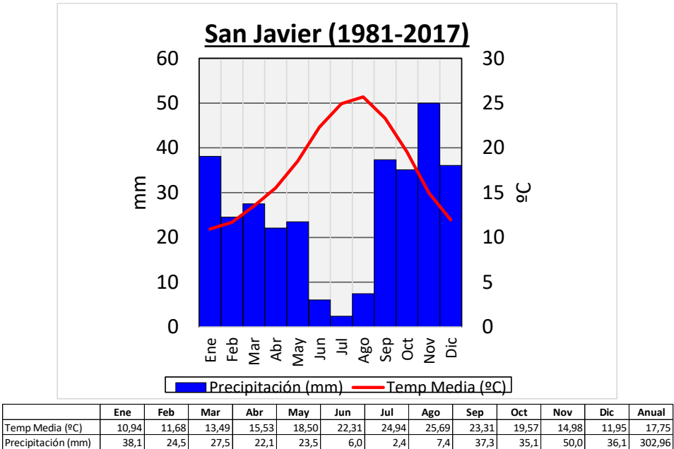
Figura 2.15. Climodiagrama de San Javier. Fuente: AEMET. Elaboración propia.
