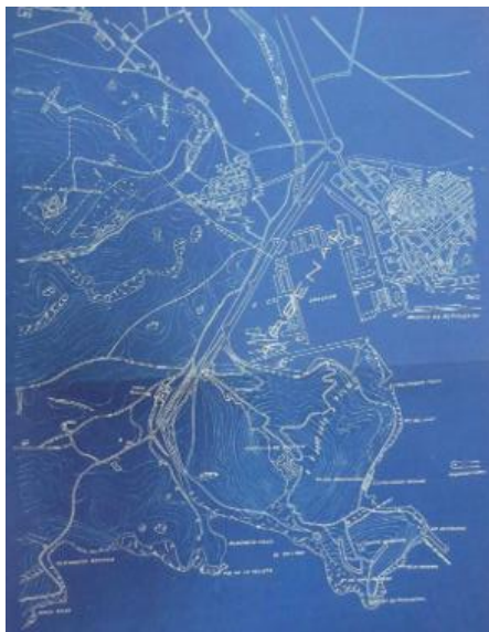
Figura 3.21. Plano general del proyecto de 1923 de depósito regulador en la Atalaya, del ingeniero Vicente Maese y jefe de Servicio Técnico Alfredo Mendizábal. Fuente: ANC, S/R PAACT A8 C45.
