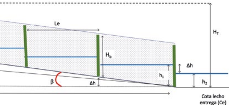
FIGURA 17 Perfil longitudinal de la rampa con indicación de las variables más representativas
