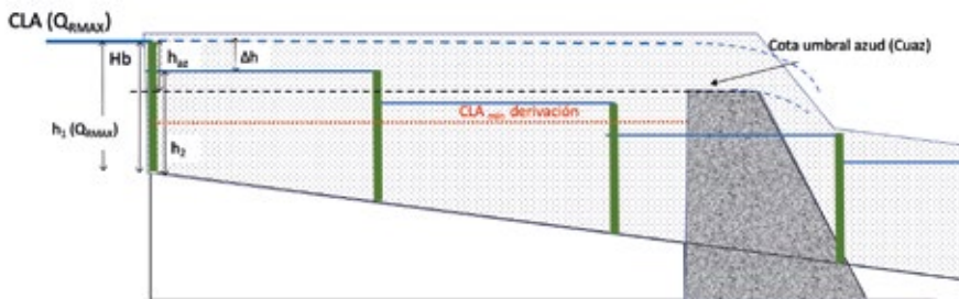
FIGURA 22 Perfil de lámina de agua cuando Qd = Q_{RMAX} + Q_{az}(h_{az})
