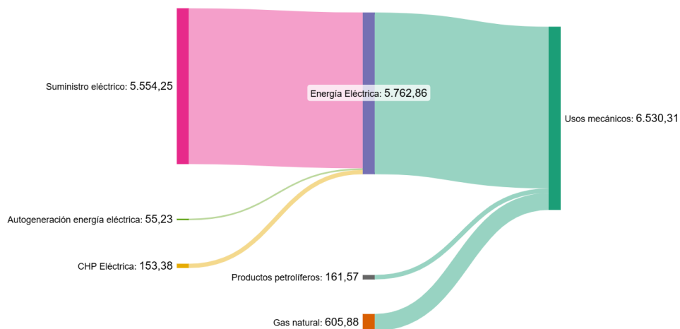
Figura 37. Distribución del consumo según fuentes de energía de los usos mecánicos (GWh) en 2021.
