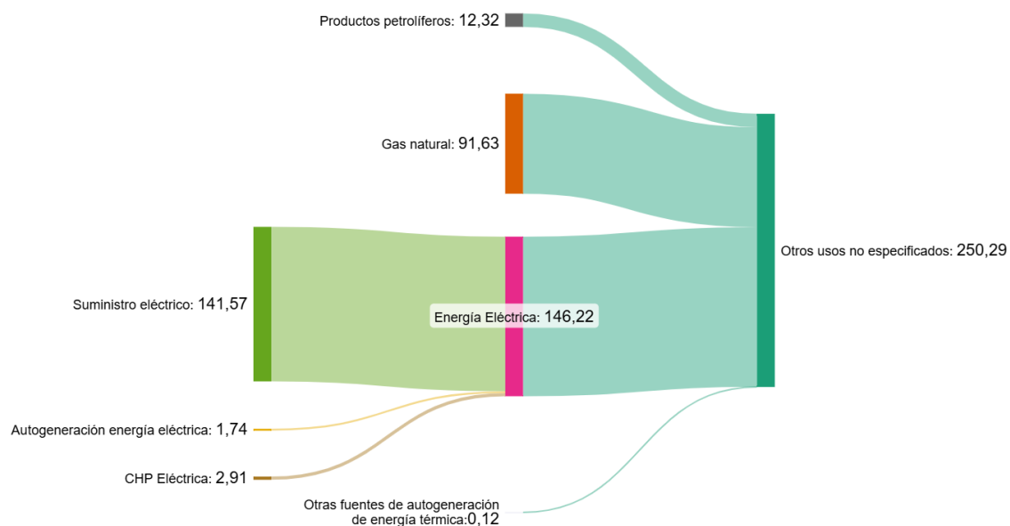
Figura 38. Distribución del consumo según fuentes de energía de otros usos no especificados (GWh) en 2021.
