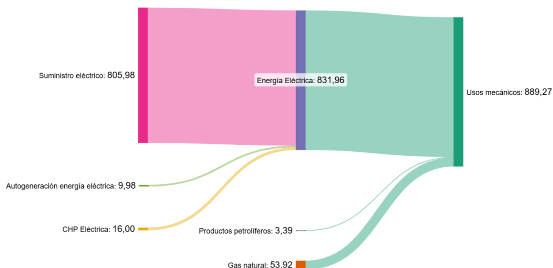
Figura 34. Distribución del consumo según fuentes de energía de los usos mecánicos (GWh) en 2021.
