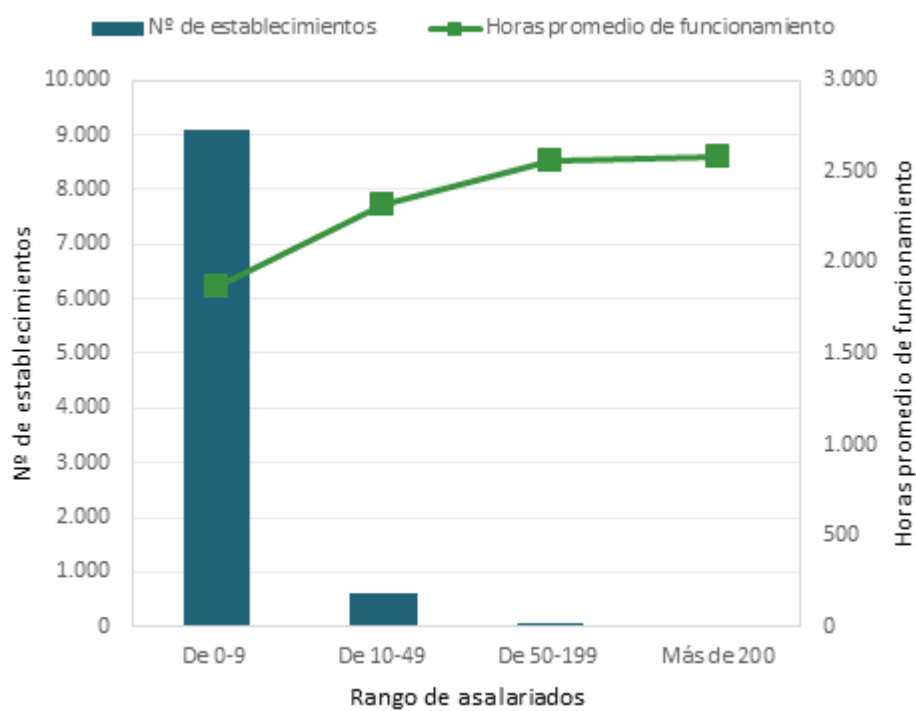
Figura 20. Horas promedio de funcionamiento anuales de las fábricas de la CNAE 14 en 2021.
