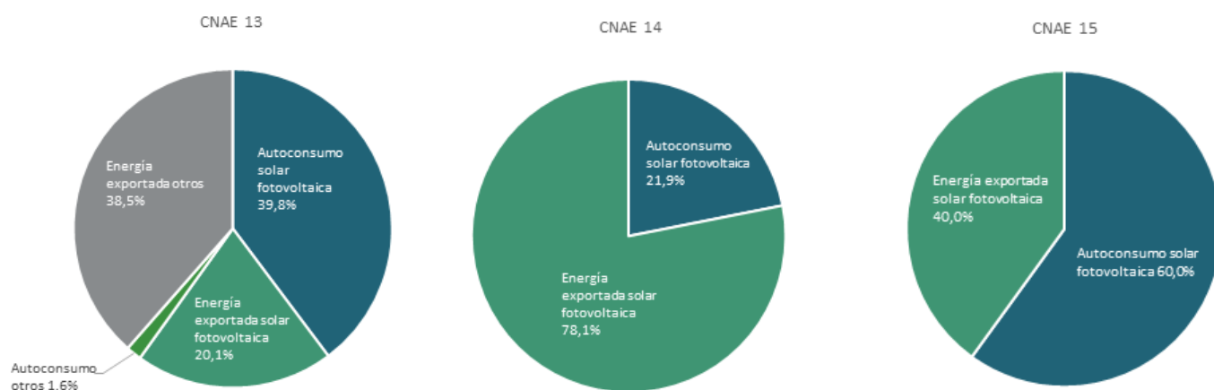
Figura 28. Distribución de energía eléctrica procedente de energías renovables y otros generadores por CNAE en 2021.
