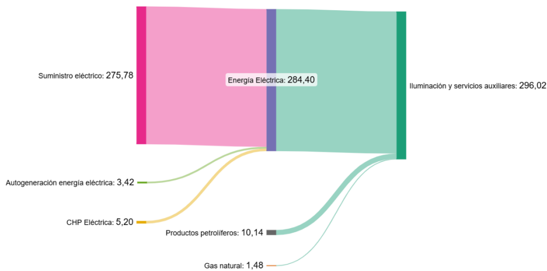
Figura 37. Distribución del consumo según fuentes de energía de la iluminación y sistemas auxiliares (GWh) en 2021.
