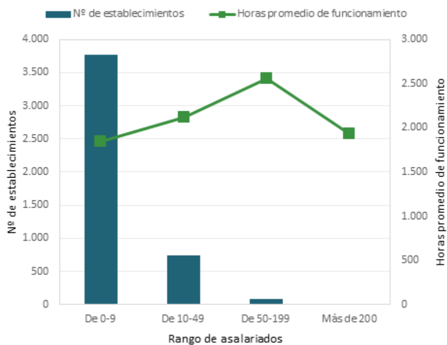
Figura 21. Horas promedio de funcionamiento anuales de las fábricas de la CNAE 15 en 2021.
