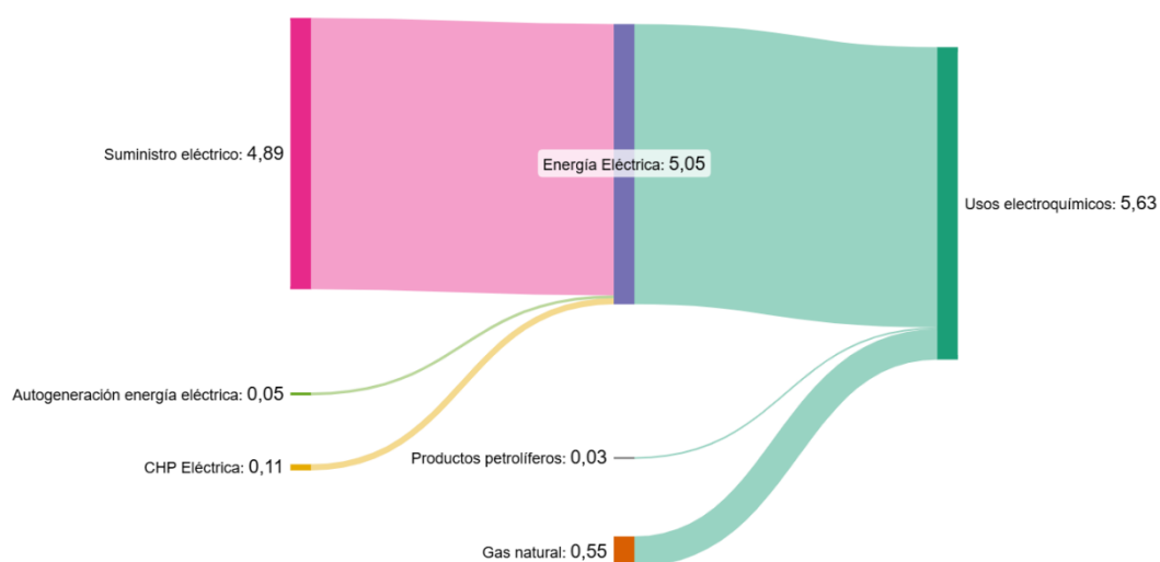
Figura 35. Distribución del consumo según fuentes de energía de los usos electroquímicos (GWh) en 2021.
