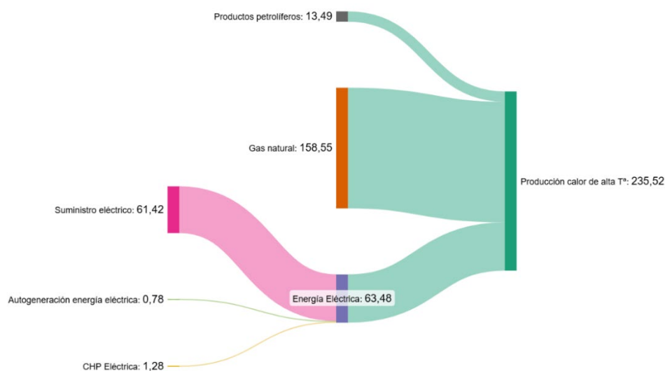
Figura 31. Distribución del consumo según fuentes de energía de la producción de calor de alta temperatura (GWh) en 2021.
