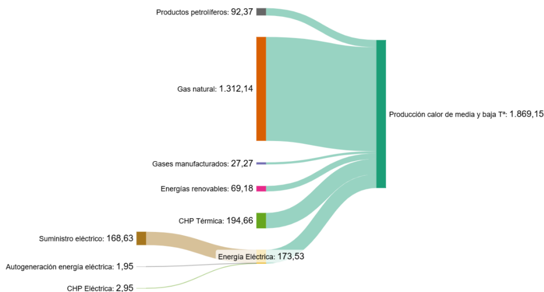
Figura 32. Distribución del consumo según fuentes de energía de la producción de calor de media y baja temperatura (GWh) en 2021.
