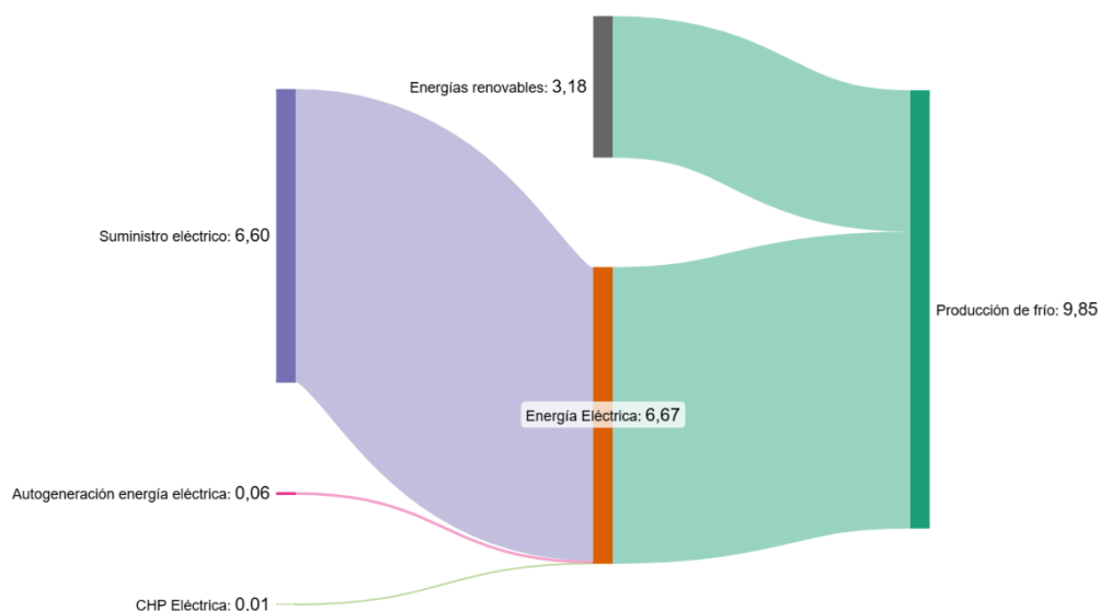
Figura 24. Distribución del consumo según fuentes de energía de la producción de frío (GWh) en 2021.
