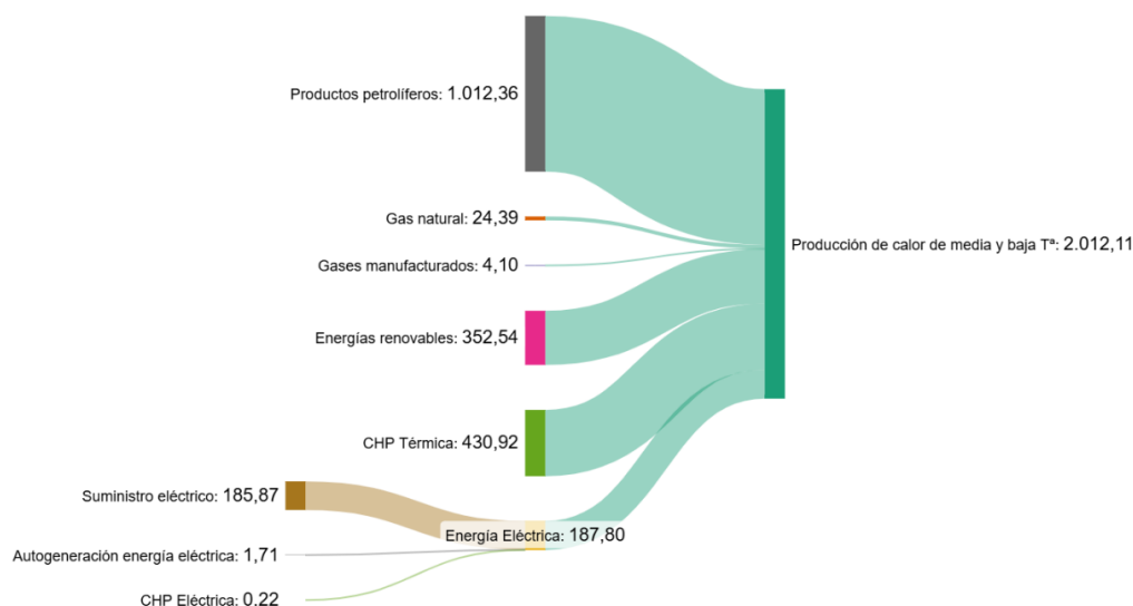
Figura 23. Distribución del consumo según fuentes de energía de la producción de calor de media y baja temperatura (GWh) en 2021.
