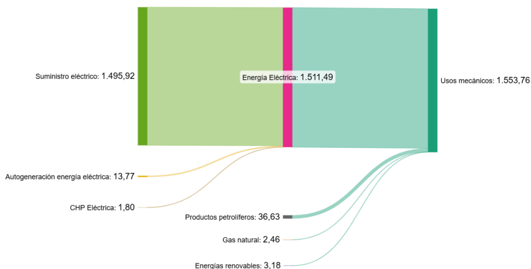
Figura 25. Distribución del consumo según fuentes de energía de los usos mecánicos (GWh) en 2021.
